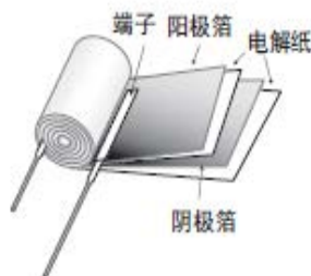
图10- 卷绕概略图
