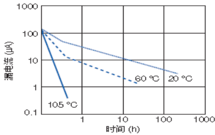
高分子固液混合电容 漏电流修复特性 100 \mu F/25 V.DC (外加 25 V.DC)
