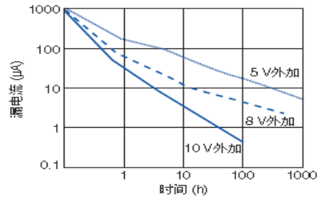
高分子固态铝电解电容器 漏电流修复特性 33 \mu F/10 V.DC (周围温度65 °C) (测定电压10V.DC)
