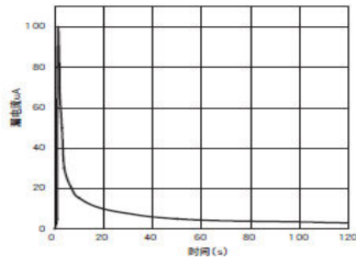
高分子固液混合电容 漏电流修复特性 100 \mu F/25 V.DC (外加 25 V.DC)
